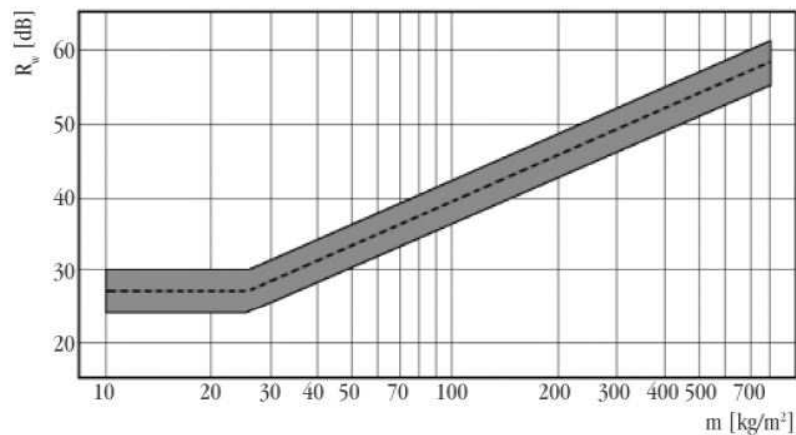
Figura 3– Índice de redução sonora em função da densidade superficial de elementos simples, homogêneos.
