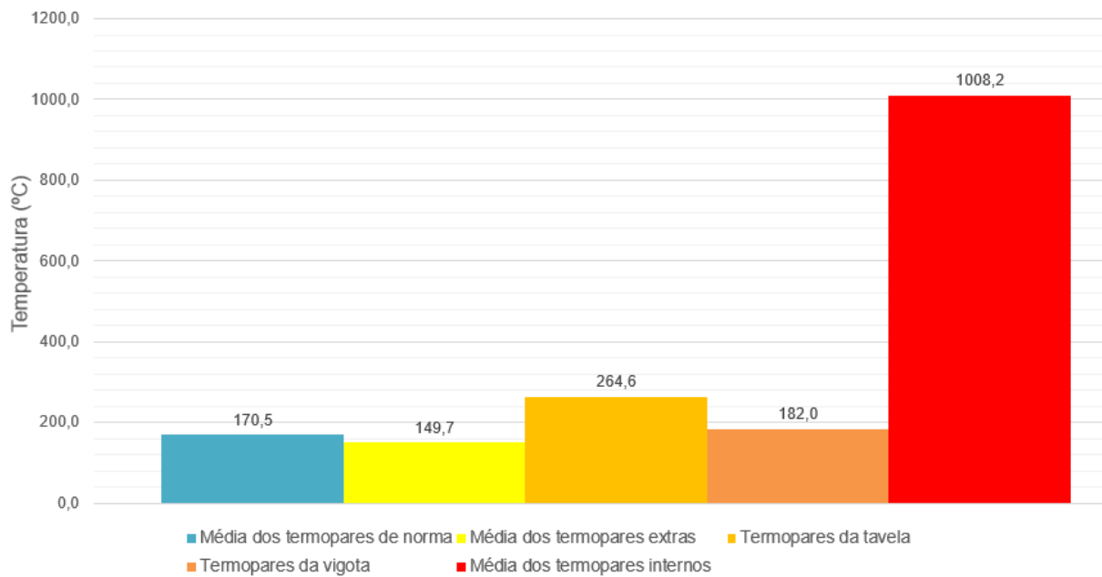
Figura 64 – Perfil de temperatura aos 134 minutos
