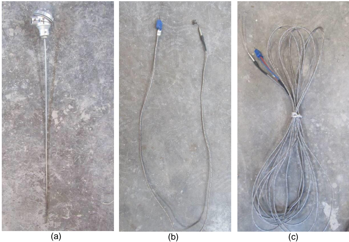
Figura 39 – Sensores de temperatura do tipo (a) K interno, (b) T externo e (c) T interno, na face da vigota e da tavela
