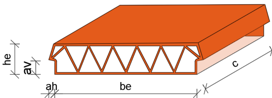
Figura 16 – Tabela cerâmica 8x37x20 cm
