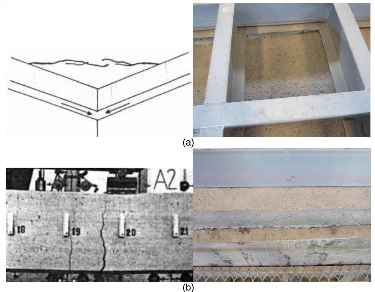
Figura 59 – Fissuras de (a) retração térmica e (b) rótula com momento fletor predominante
