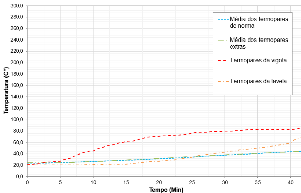
Figura 54 – Temperatura em relação ao tempo de ensaio
