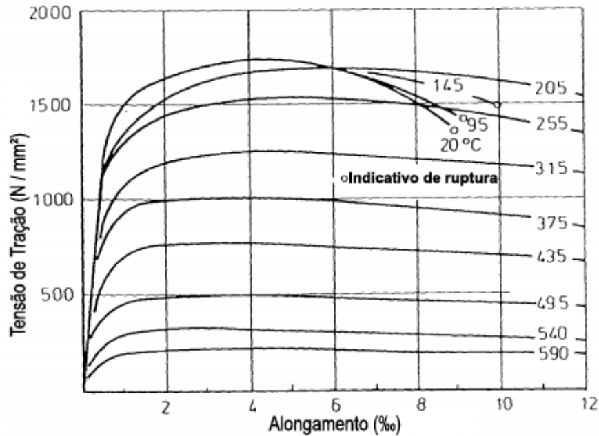
Figura 11 – Tensão-deformação relacionada a temperatura para aço de protensão
