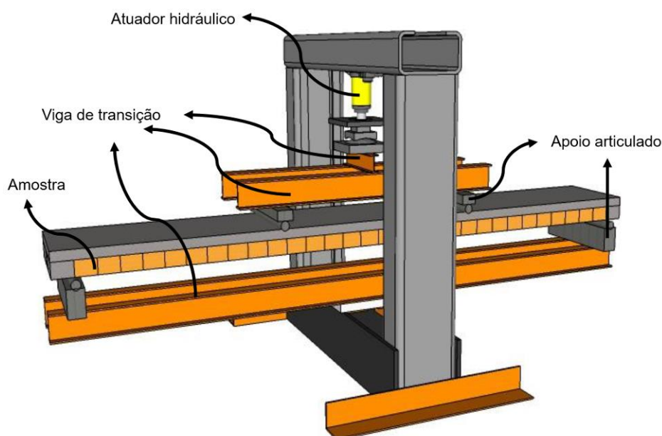
Figura 32 – Esquema do ensaio da LA1
