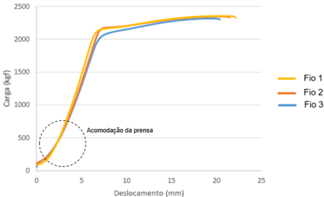
Figura 18 – Gráfico de carga por deslocamento dos fios de \varnothing = 4\text{mm}
