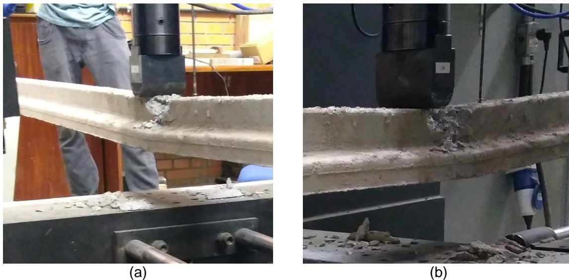
Figura 71 – Forma de ruptura da vigota (a) LP1 V1 e (b) LP2 V1
