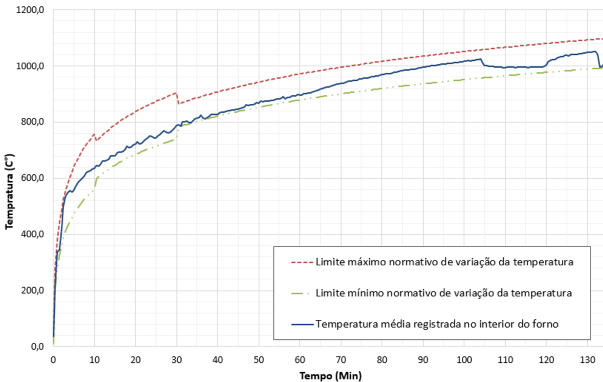
Figura 66 – Curva do ensaio para 134 minutos
