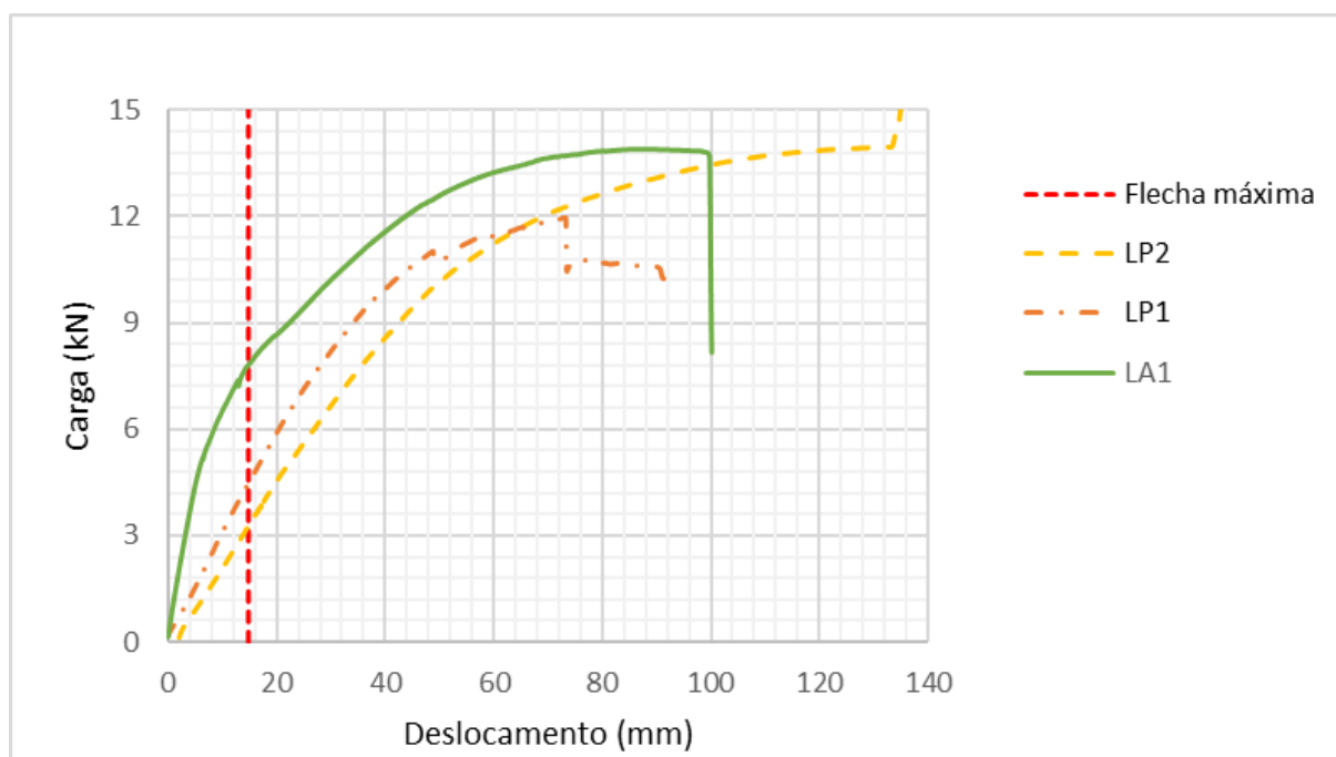
Figura 75 – Comparativo entre nervuras
