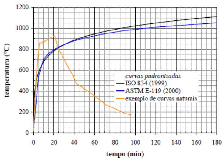
Figura 9 – Curvas de incêndio padrão normalizadas
